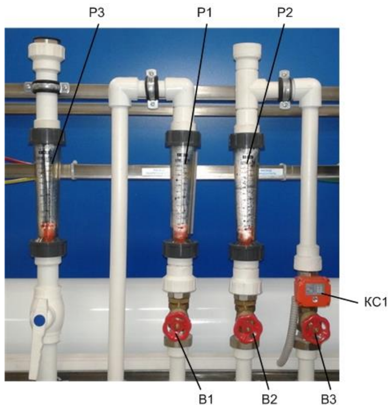
Рис.3 Ротаметры и вентили
