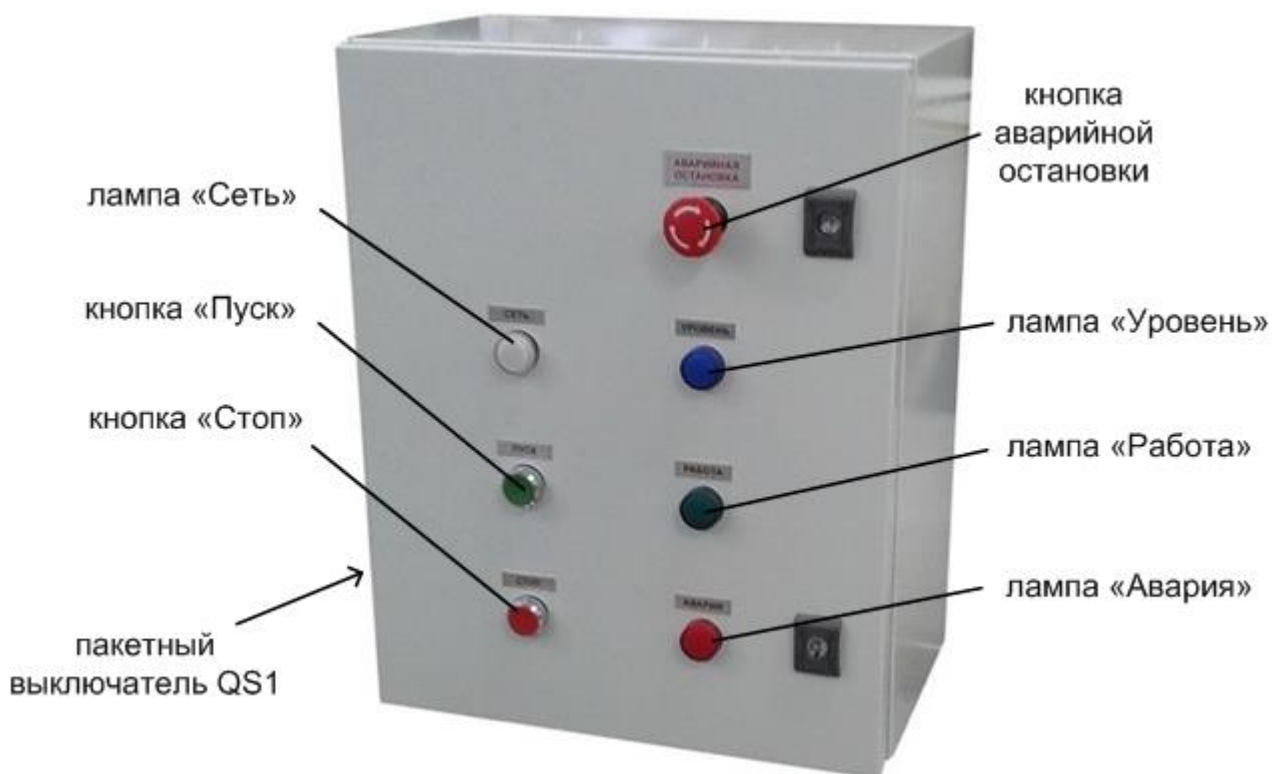
Рис.4 Блок управления.
