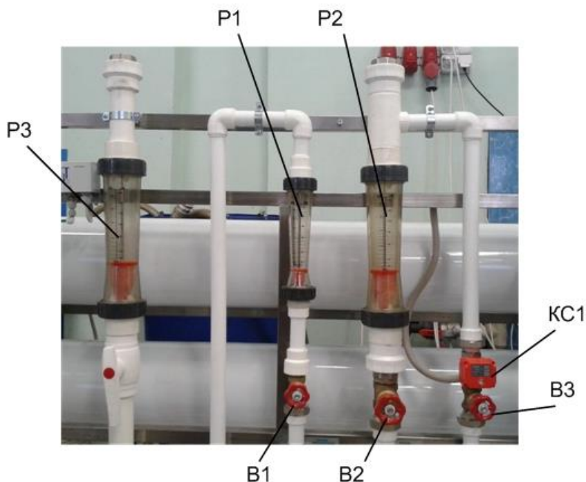
Рис.3 Ротаметры и вентили
