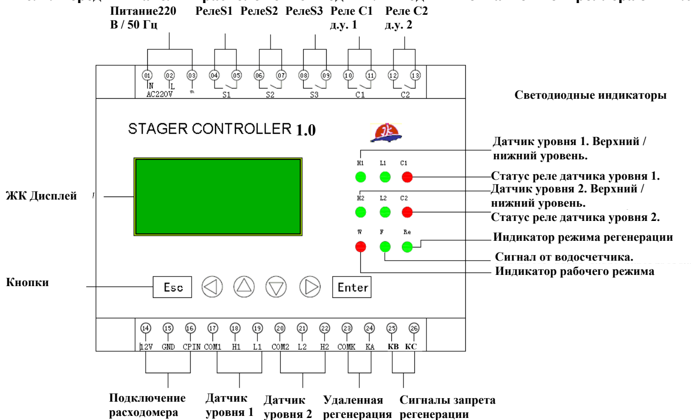
Рис. 1. Передняя панель и расположение входных/выходных контактов контроллера ЖКА1.0
