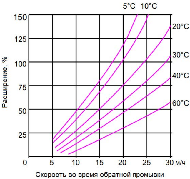
Расширение слоя во время обратной промывки
