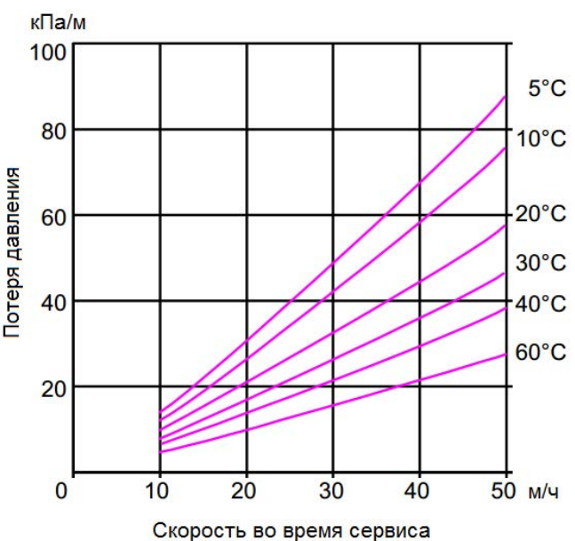
Потери давления
